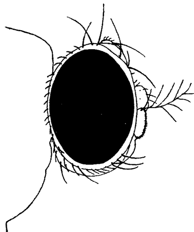
FIG. 46.— Drosophila simulans .
