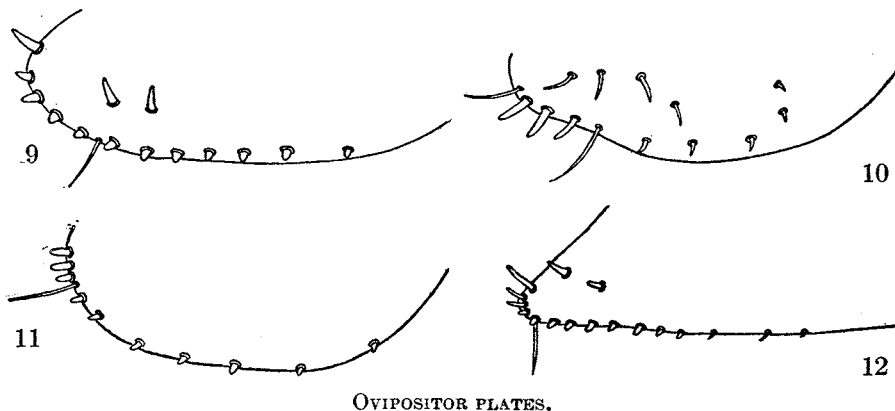
FIG. 9.— Scaptomyza adusta .
